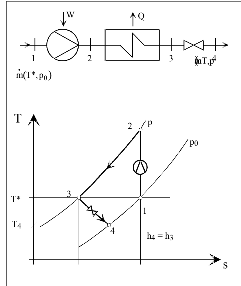
Fig. 13: Offener Prozess nach Claudé zur Kühlung eines Gasstromes mit Umgebungstemperatur \dot{m}(T^*, p_0) durch Kompression (1 → 2), Kühlung (2 → 3) und nachfolgende Expansion in einer Drossel (3 → 4) auf die Temperatur ( T_4 < T^* ). Fließbild und Temperatur ( T ) – Entropie ( S ) – Diagramm [36].
